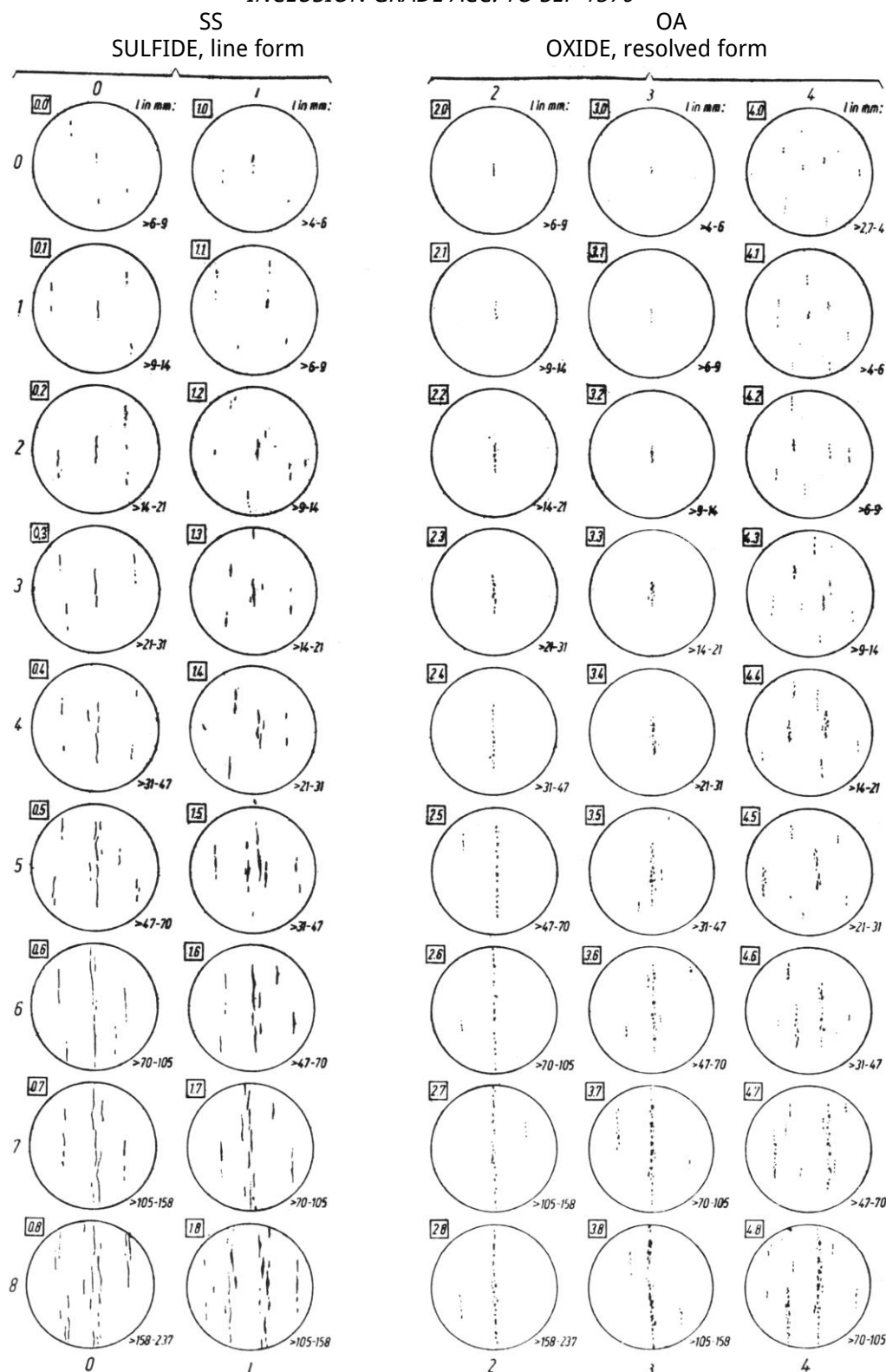
Figura 534 - Immagini tipo per la valutazione delle inclusioni secondo UNI 3244/80 o SEP 1570 (ridotte a circa un terzo rispetto alle originali)
